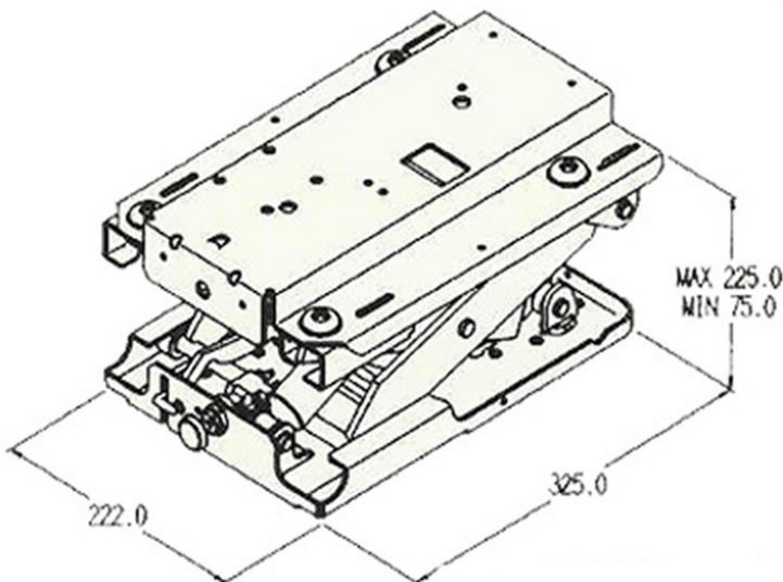
Pneumatique KAB 15
